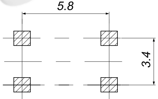
印制线路板 Recommended P.C.B layout
